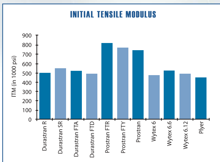
INITIAL TENSILE MODULUS (average values in kpsi)
